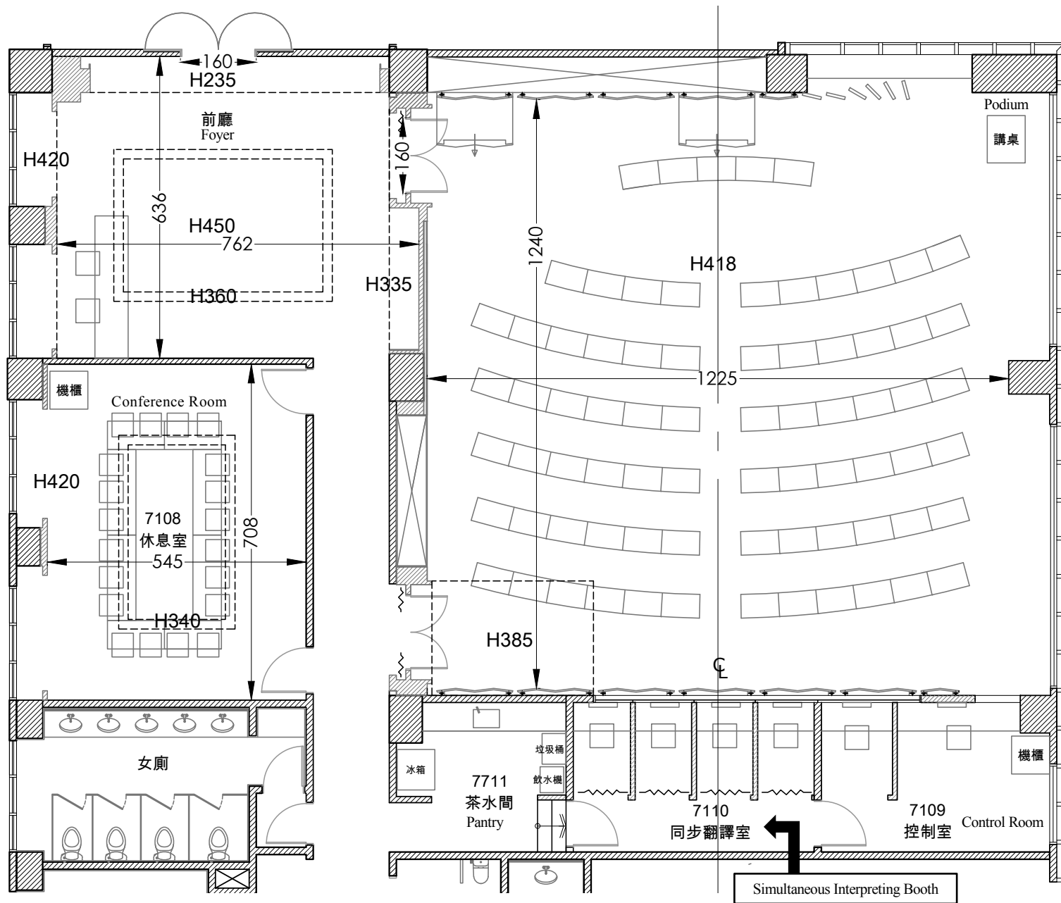
圖 (一) 國際會議廳_平面圖 (單位: 公分) Figure(1) International Conference Hall_Floor Plan (Unit: cm)
